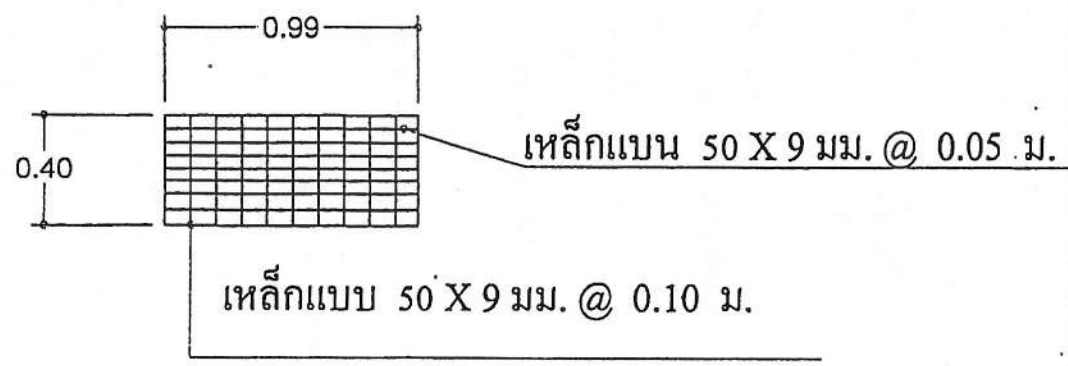
แบบฝาตะแกรงเหล็ก
