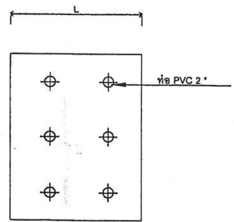
แบบขยายฝาบ่อพัก ท่อ Ø 1.20 ม. มาตรฐาน 1:25
